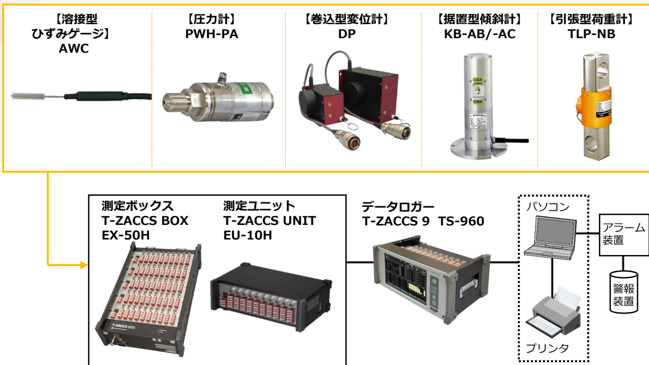
【システムブロック図】
