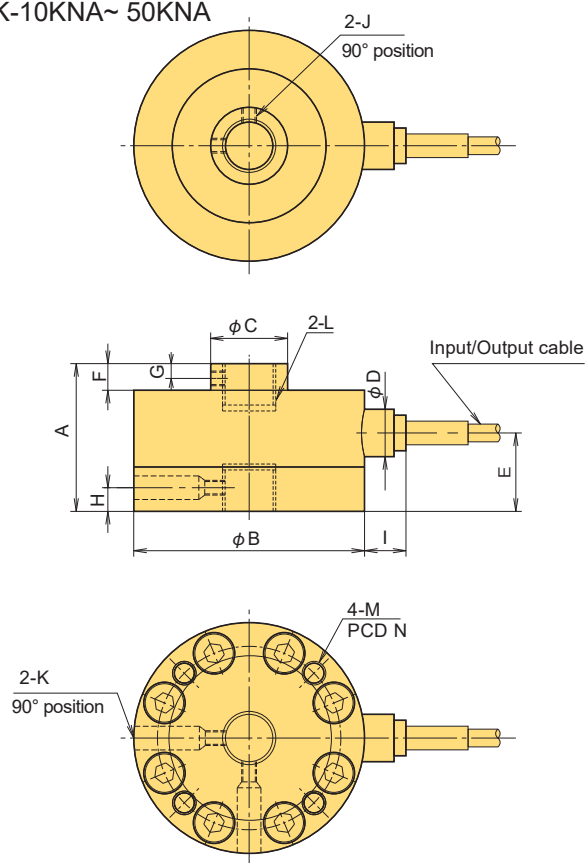
TCLK-10KNA~ 50KNA
