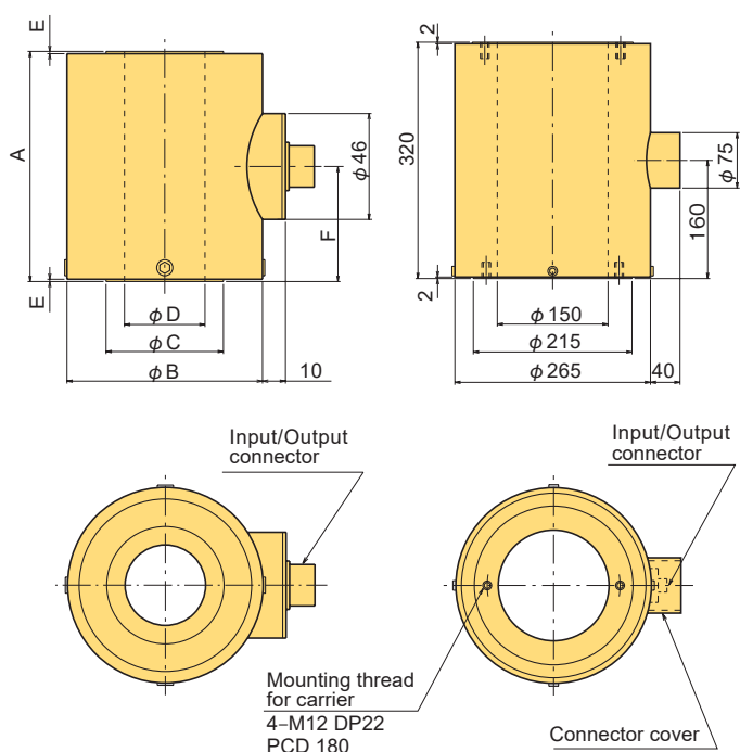
CLC-50KNA~ 3MNA
