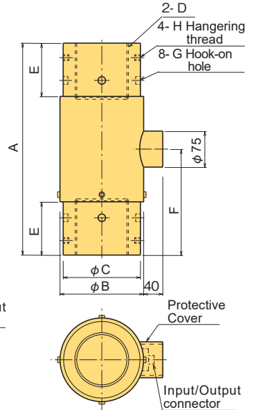
TCLP-1 ~ 2MNB
