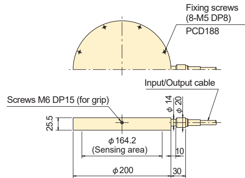
KDJ-PA
